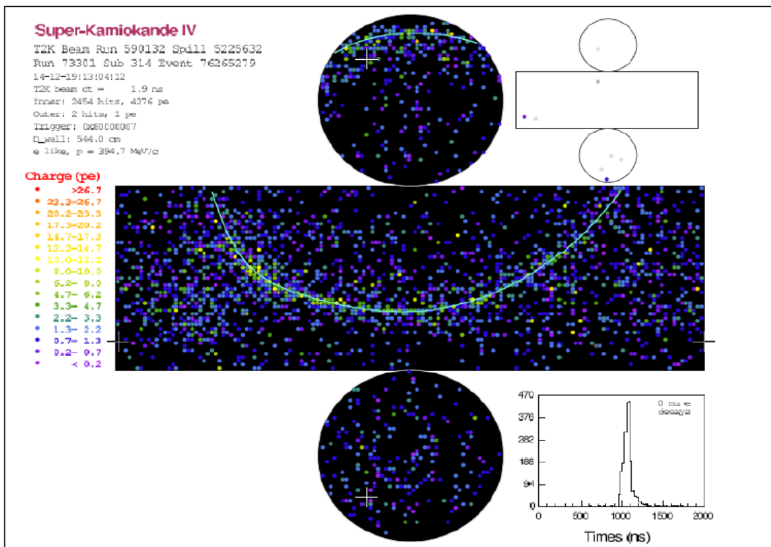
Рис.3. Электронное антинейтрино, зарегистрированное в детекторе СуперКамиоканде.
